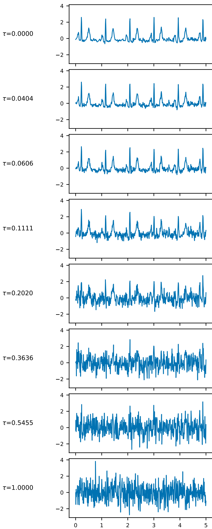
Diffusion
